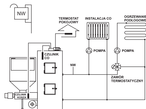
Rys.5. Sterowanie kotłem podajnikowym z jednym obiegiem grzewczym sterowanym termostatem pokojowym, ogrzewaniem podłogowym sterowanym zaworem termostatycznym.
